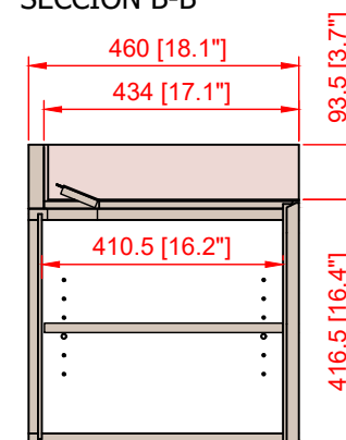
SECCIÓN B-B'
