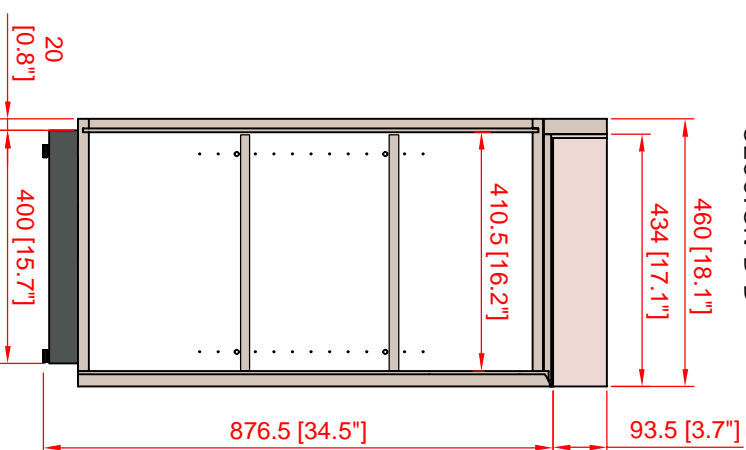
SECCIÓN B-B'
