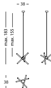
Suspensión cable
