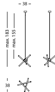
Suspensión rígida
